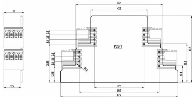
PC BOARD LAYOUT DIMENSIONI CIRCUITO STAMPATO
